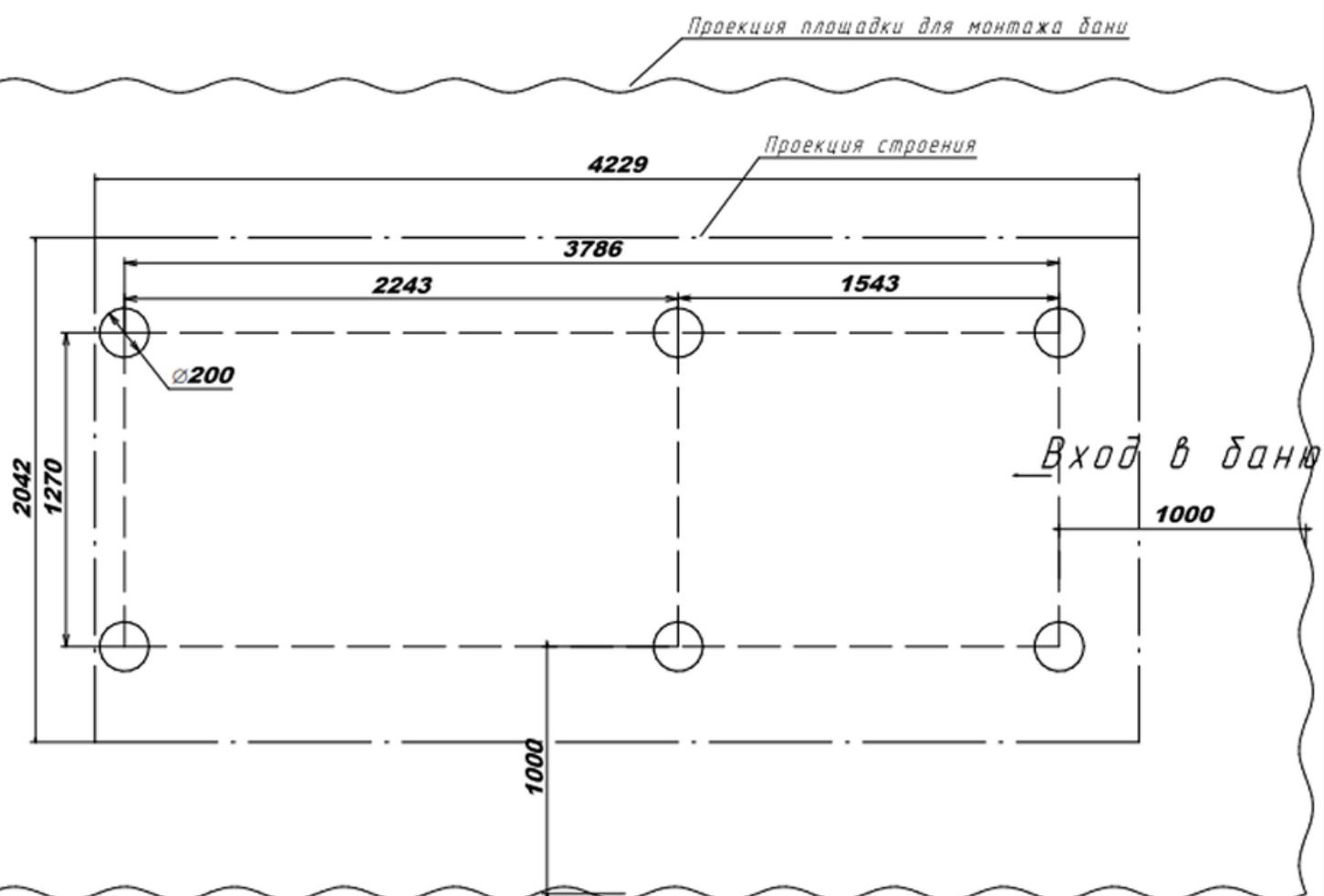
Чертеж свайного фундамента для бани-бочки с 2-я помещениями
