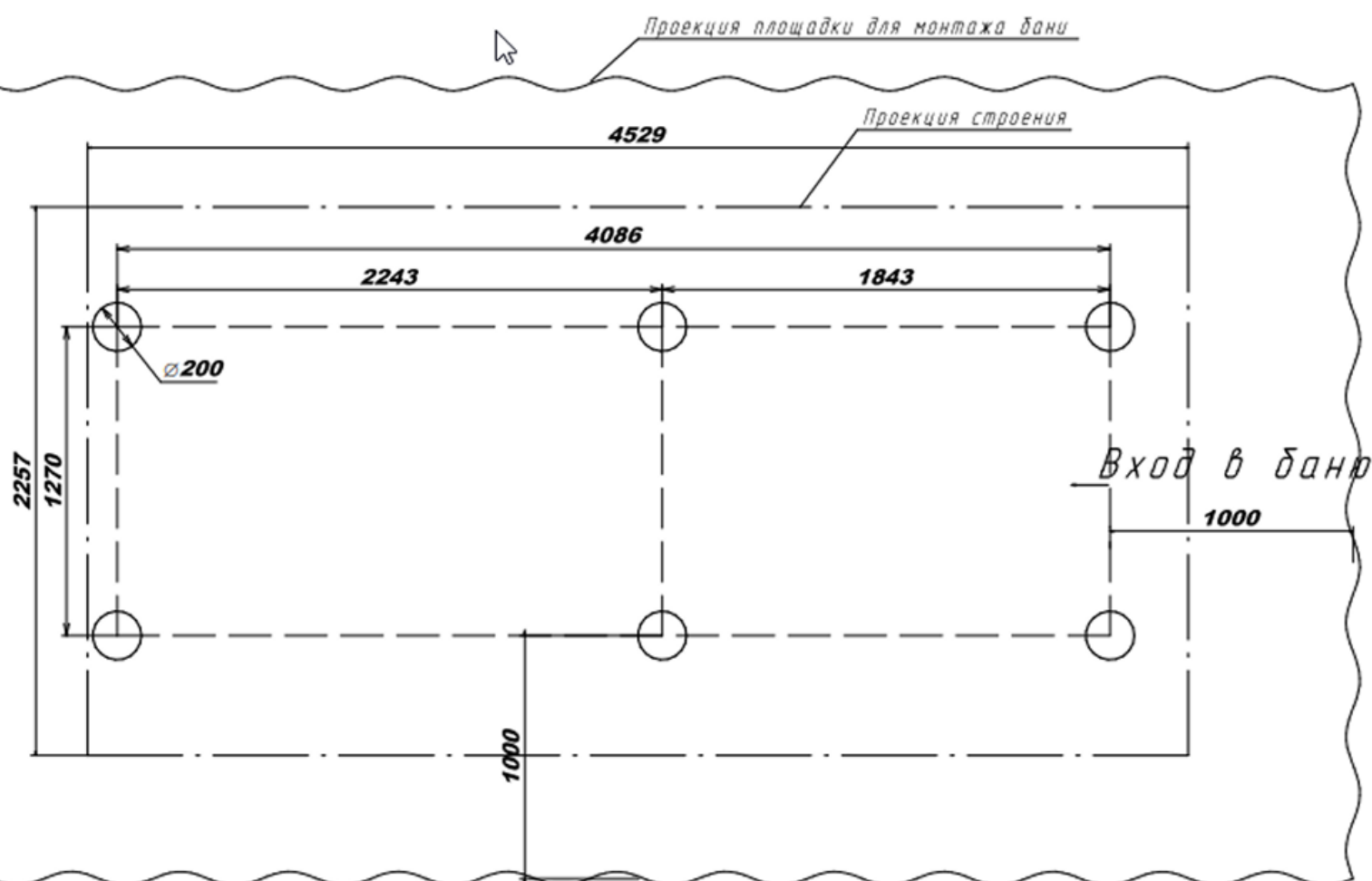
Чертеж свайного фундамента для бани-бочки с 2-я помещениями
